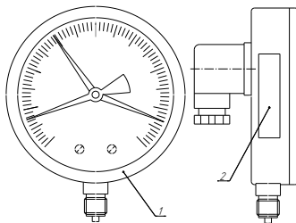
1 - манометр ЭЖМ, 2 - табличка
